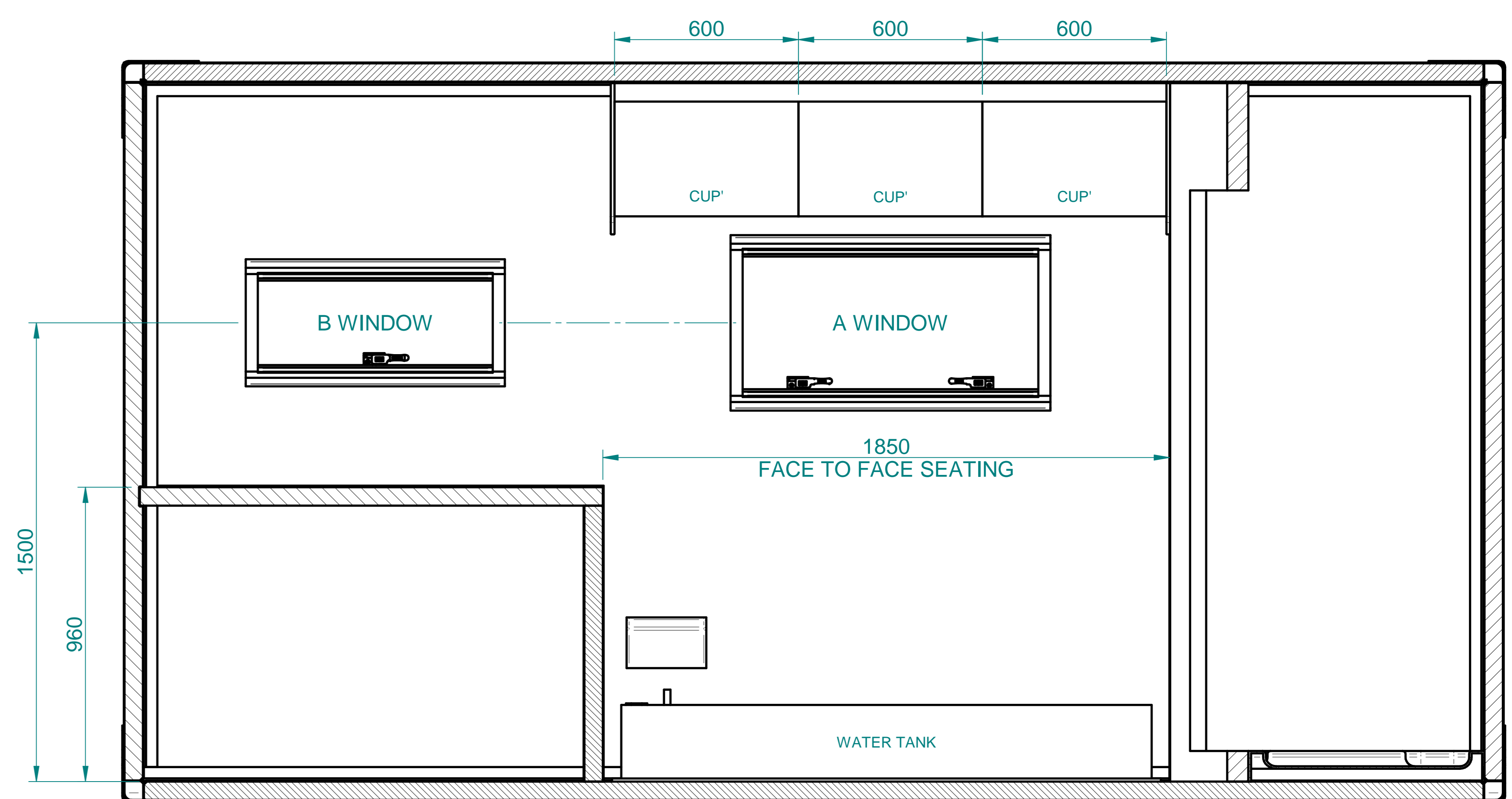
SECTION A-A 1:10
